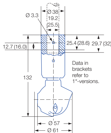
Slip-on connection ASME - BPE 1997 (OD-Tube)
