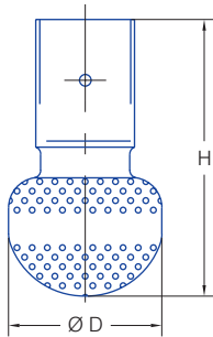
Slip-on connection ASME - BPE 1997 (OD-Tube)
